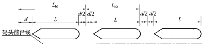
图 4.4.2-2 多个泊位长度
